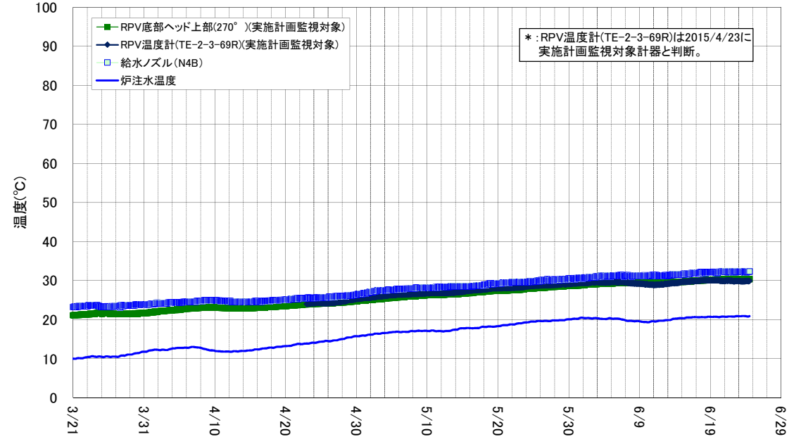
2号機 原子炉压力容器まわり温度(3/21~6/29)
