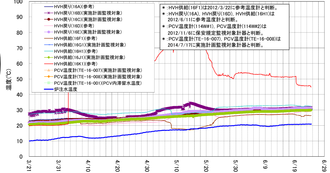
2号機 D/W雰囲気温度(3/21~6/29)
