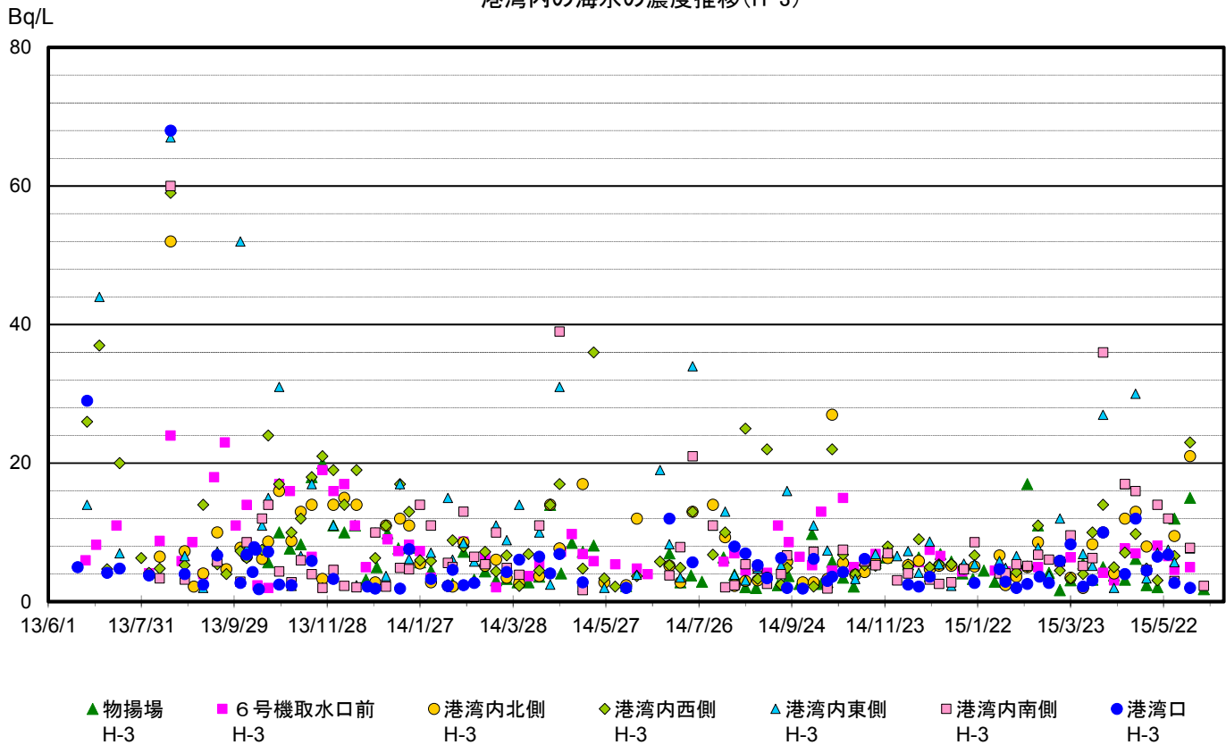
港湾内の海水の濃度推移(H-3)
