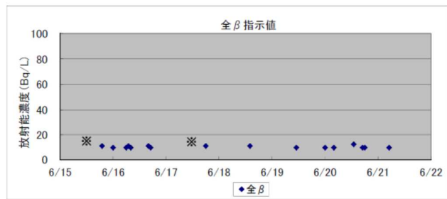
港湾口海水放射線モニタ指示値 (2015年6月15日 ~ 6月21日 分)
