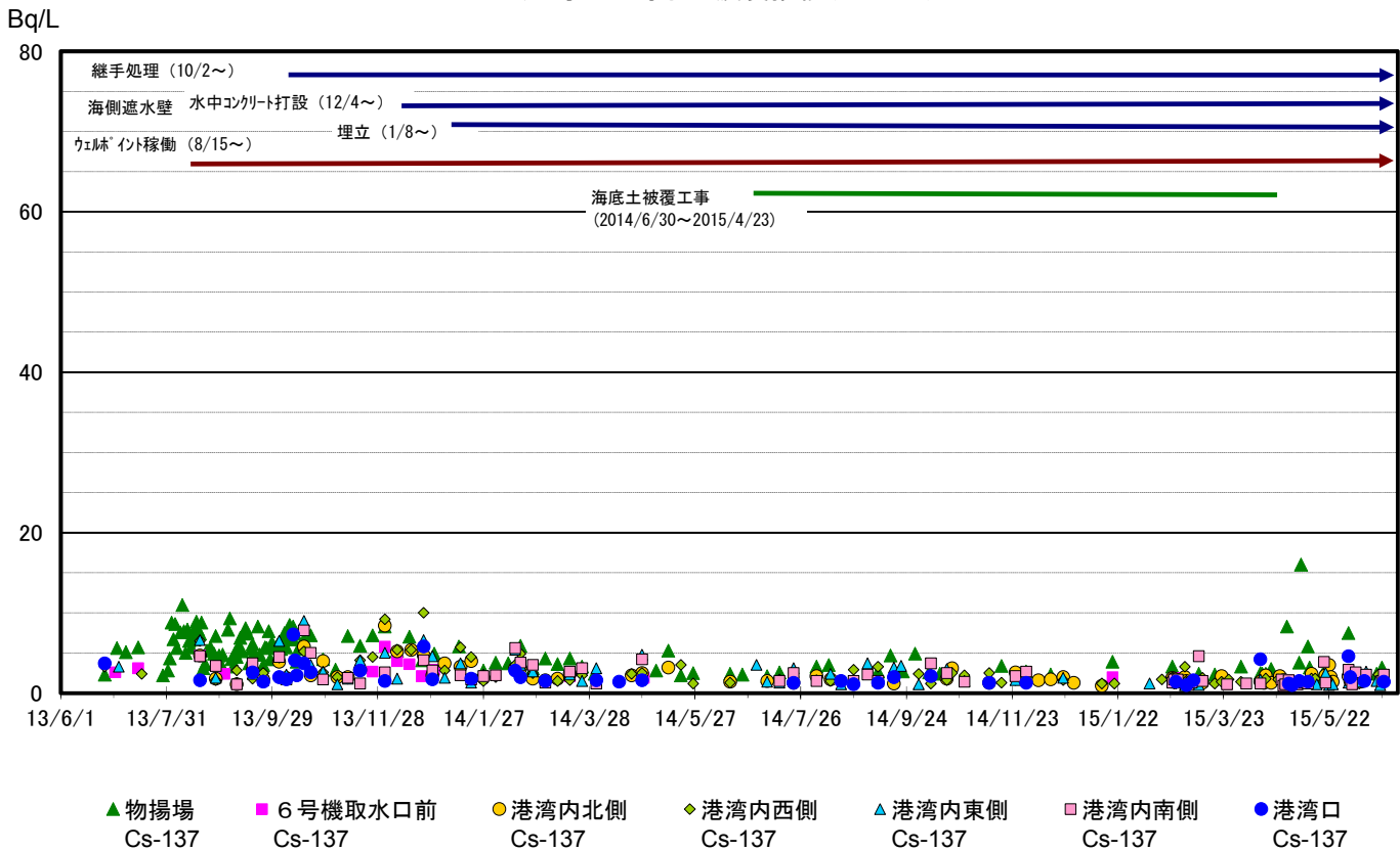
港湾内の海水の濃度推移(Cs-137)
