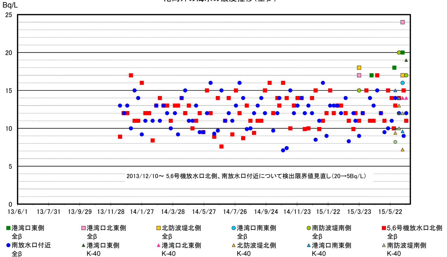
港湾外の海水の濃度推移(全β)
