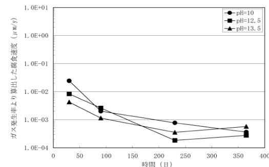
図2 ガス発生試験のイメージと金属腐食速度の例
