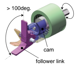
高精度立体カム機構
