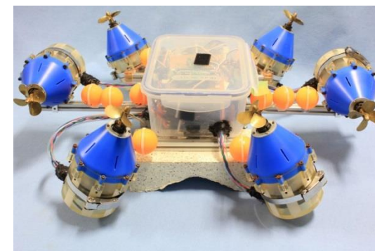
試作した水中移動ロボット
