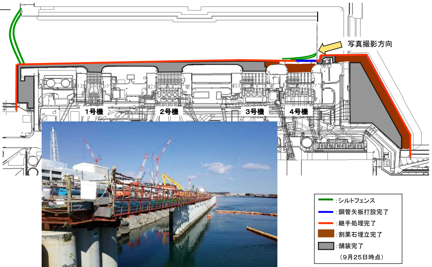
海側遮水壁閉合箇所 : 鋼管矢板9本分(延長約10m)
