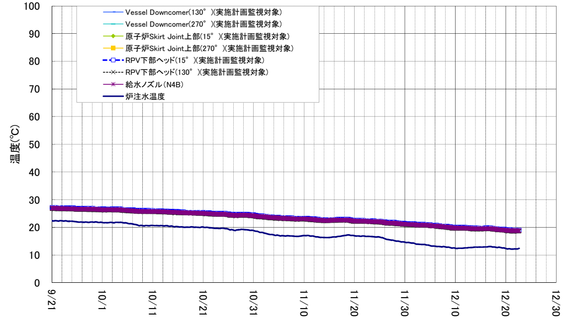
1号機 原子炉压力容器まわり温度(9/21~12/22)
