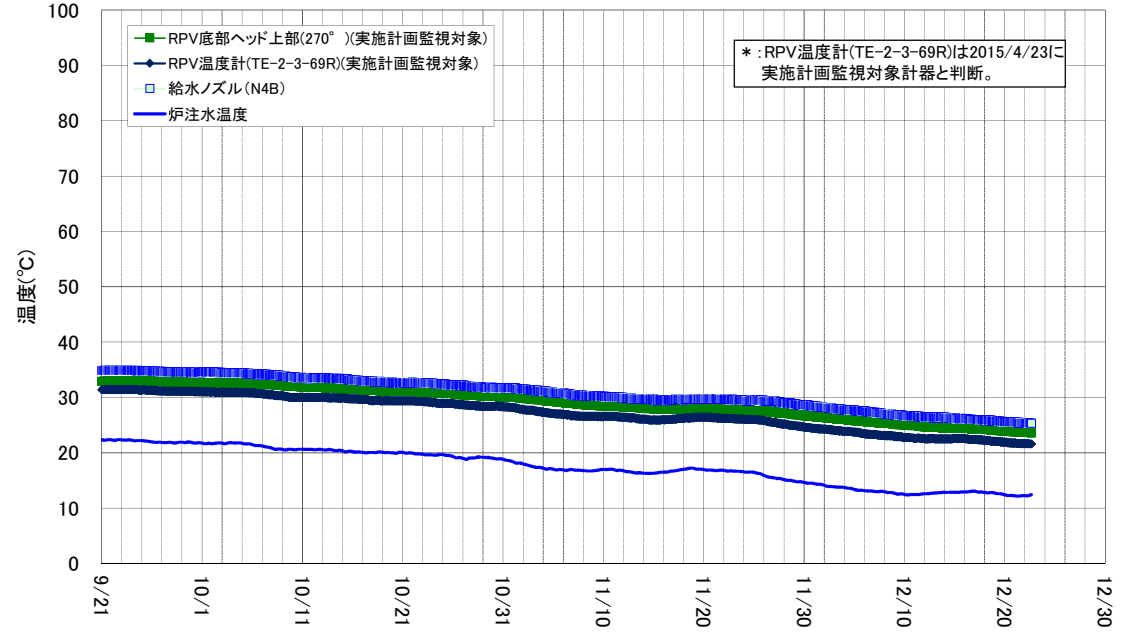
2号機 原子炉压力容器まわり温度 (9/21~12/22)
