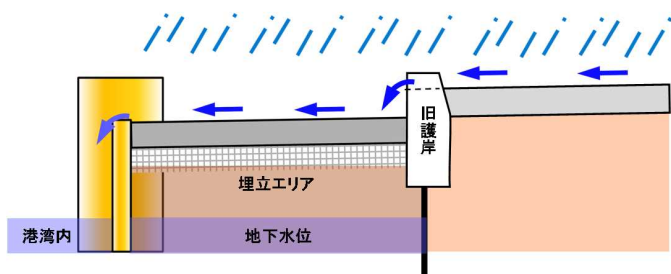
遮水壁閉合前
