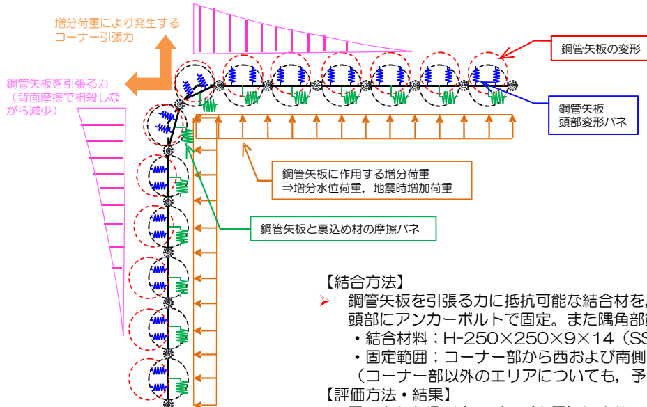
<コーナー部における梁ハネモデル>
