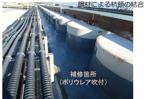
鋼管矢板際の状況（補修実施後） （ポリウレタ吹付箇所の一例）
