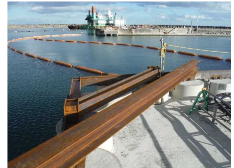
【コーナー部における杭頭結合状況】
