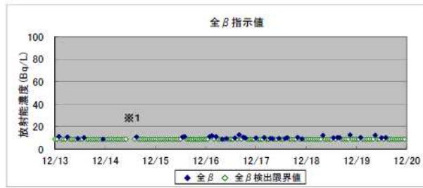
港湾口海水放射線モニタ指示値 (2015年12月13日 ~ 12月19日 分)
