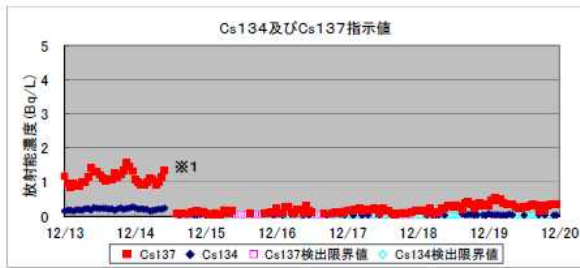
港湾口海水放射線モニタ指示値 (2015年12月13日 ~ 12月19日 分)
