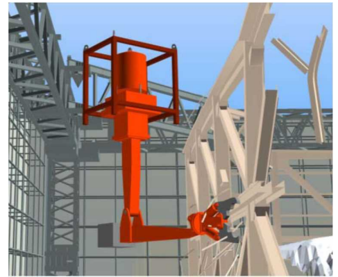
支障となる鉄骨の切断イメージ
