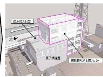
燃料取り出し用カバーの設置
