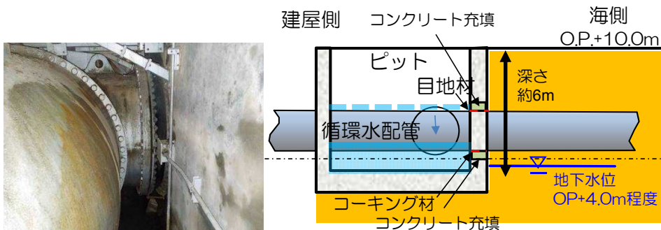
逆洗弁ピット配管接続部付近断面図
