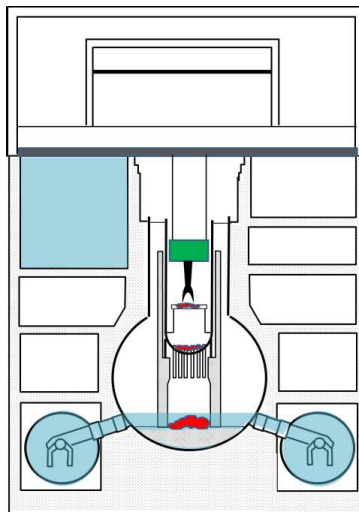
b. 気中-上アクセス工法
