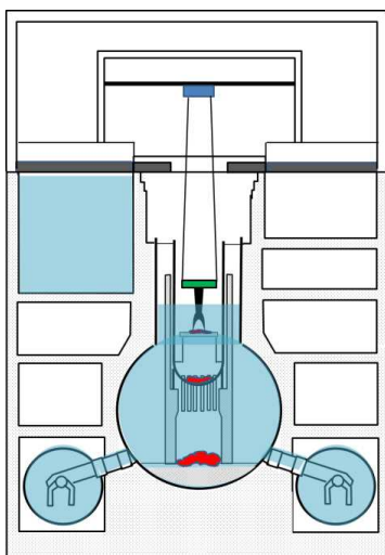
a. 冠水-上アクセス工法
