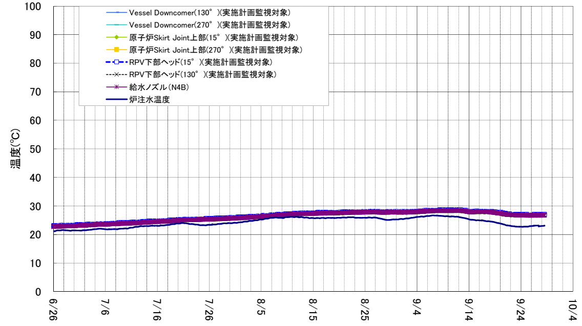
1号機 原子炉压力容器まわり温度(6/26~9/28)
