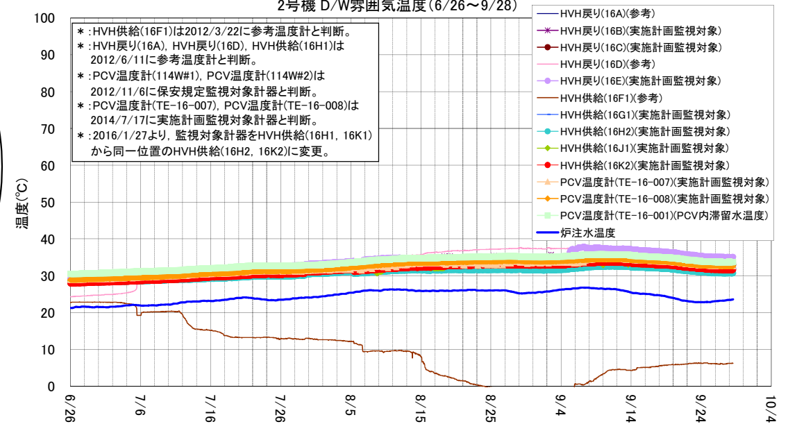
2号機 D/W雰囲気温度 (6/26~9/28)
