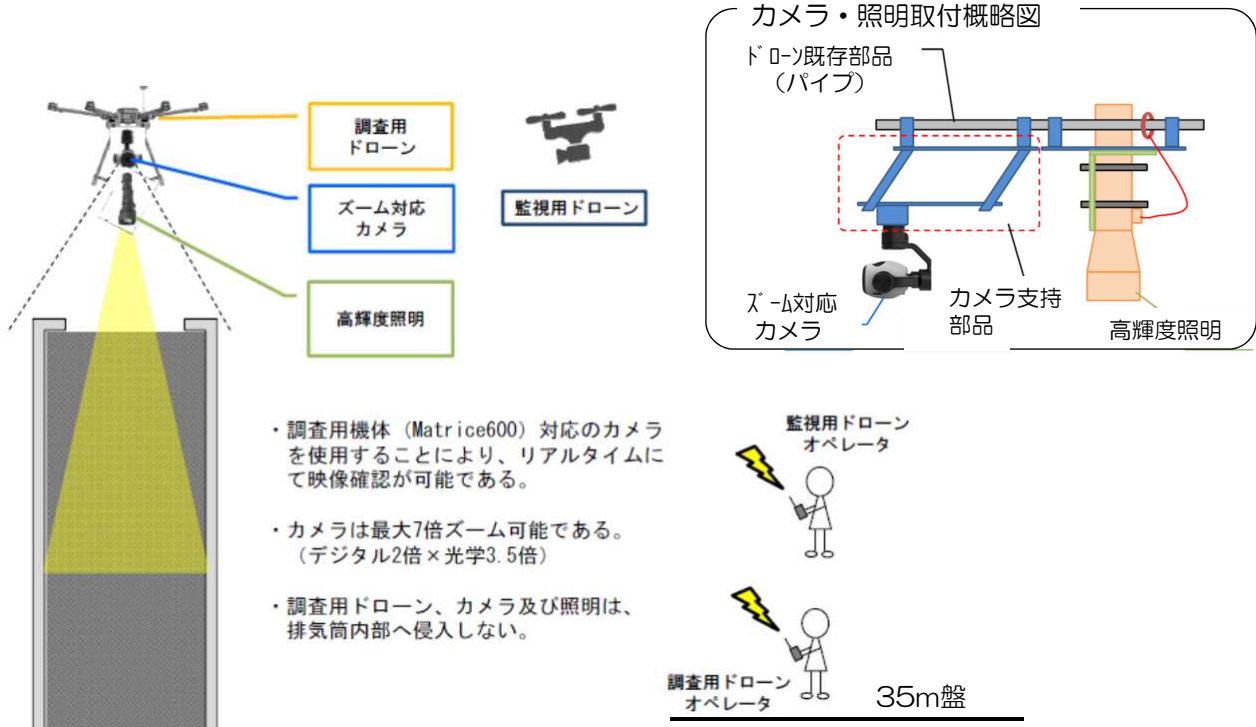
ズーム機能付きカメラを使用した調査方法のイメージ
