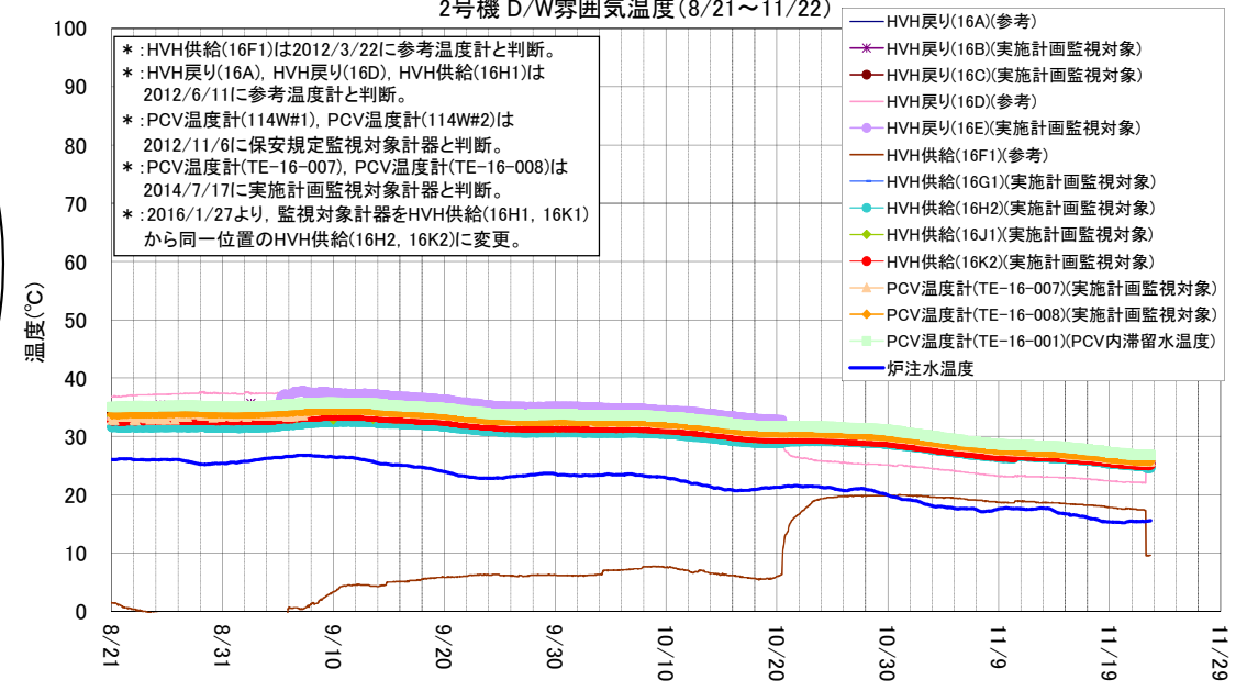
2号機 D/W雰囲気温度(8/21~11/22)
