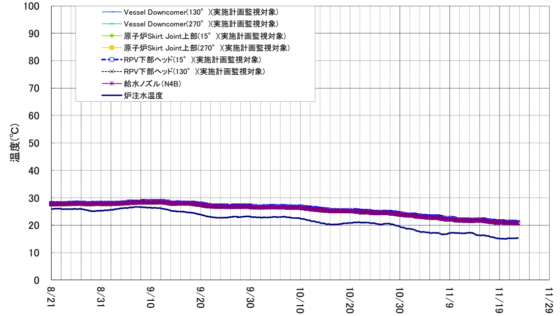
1号機 原子炉压力容器まわり温度(8/21~11/22)
