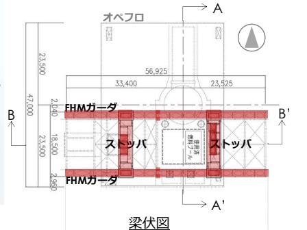
梁伏図
