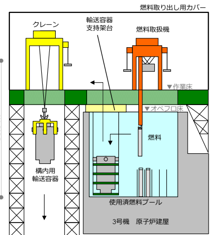
3号機燃料取り出し作業イメージ
