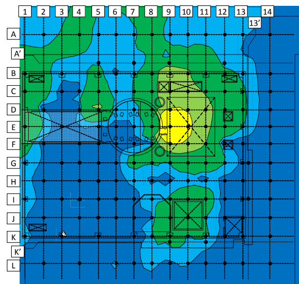
全遮へい体設置後※ (2016.12.5~12.15測定)
