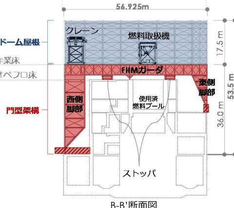
B-B'断面図
