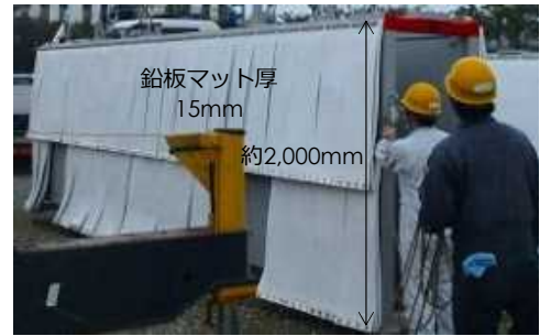
衝立形状④
