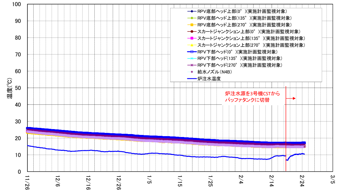
3号機 原子炉圧力容器まわり温度(11/26~2/24)
