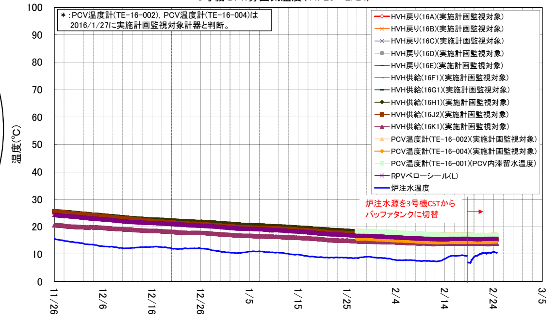
3号機 D/W雰囲気温度(11/26~2/24)
