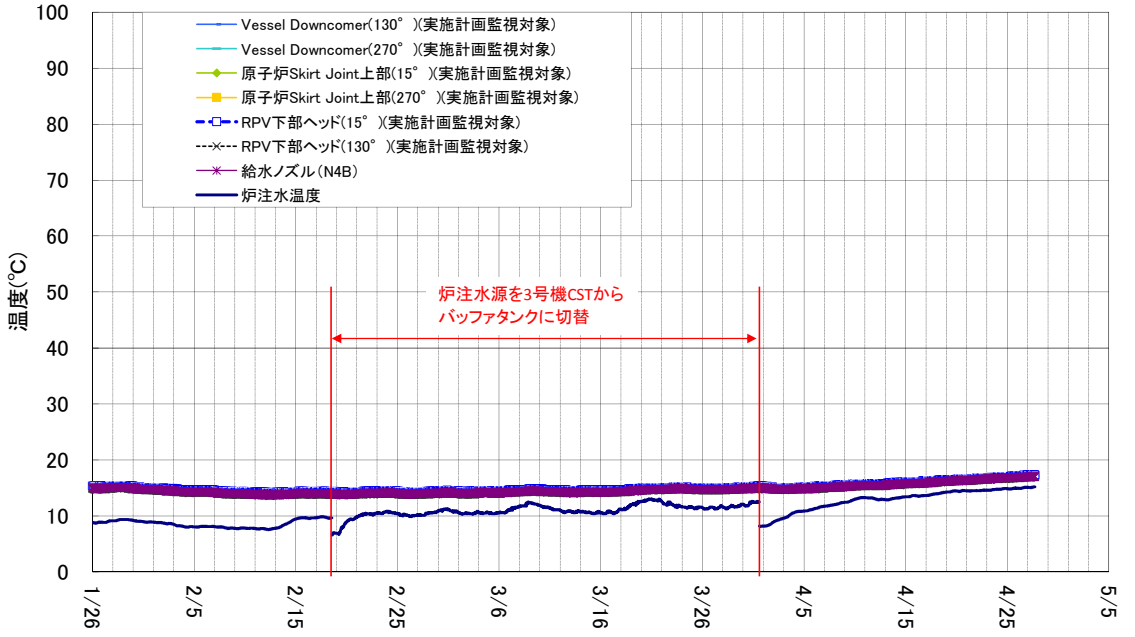
1号機 原子炉圧力容器まわり温度(1/26~4/27)
