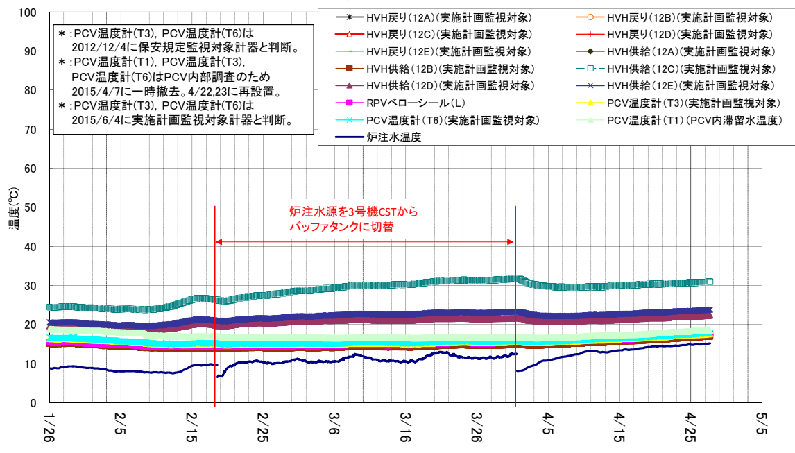
1号機 D/W雰囲気温度(1/26~4/27)
