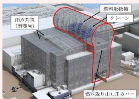
燃料取り出し用カバーイメージ
