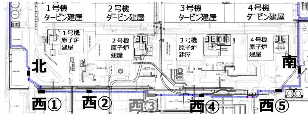
■ : 補助工法対象箇所 ■ : 未凍結箇所
