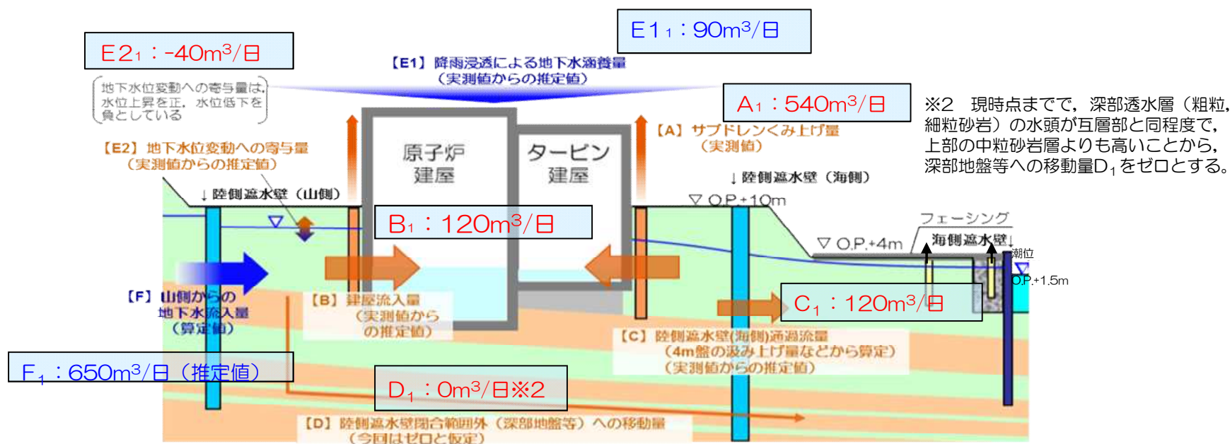
実測に基づく地下水収支の評価 (2017.3.1~3.31)
