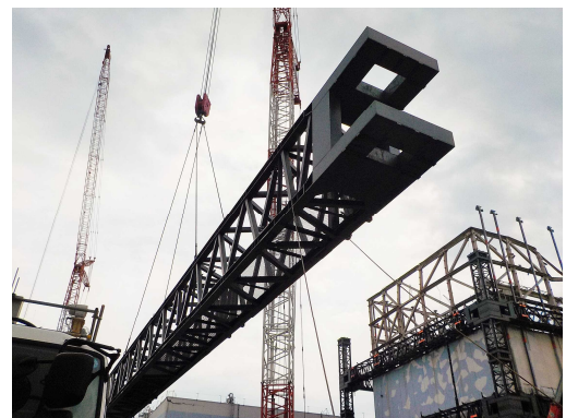
柱・梁取り外し （中段南梁）
