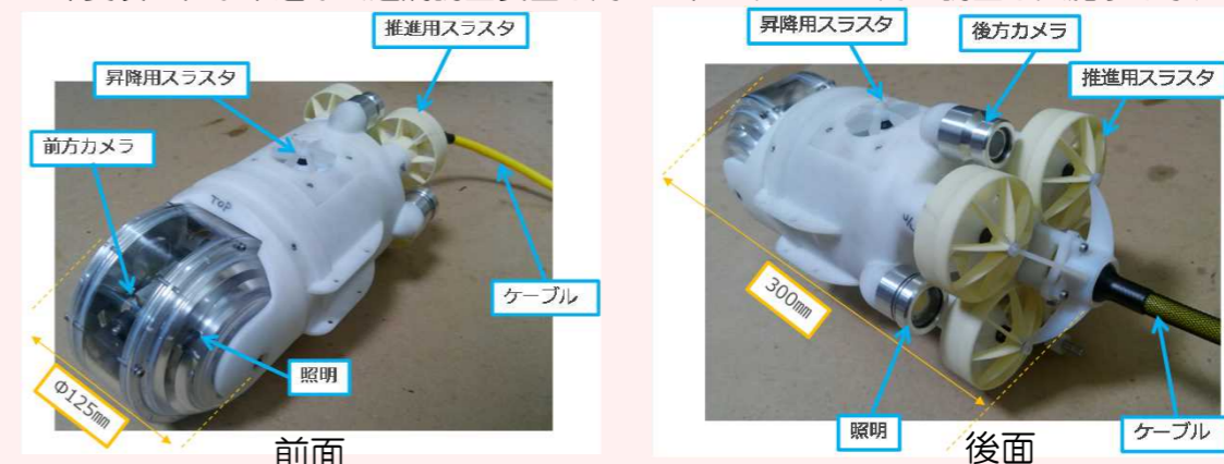
水中遊泳式遠隔調査装置
