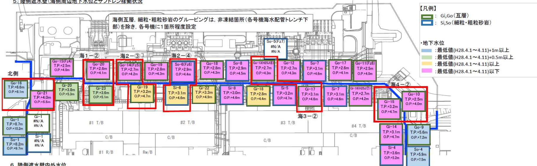
陸側遮水壁運用における監視項目(海側 互層、細粒・粗粒砂岩水位)
