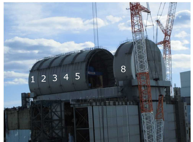
3号機原子炉建屋オペフロ全景 (12月19日時点)
