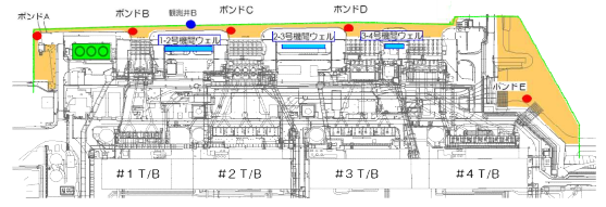
サブドレン集水タンク及びT/B移送量 (m³/日週平均)
