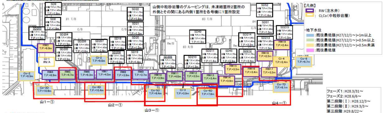
陸側遮水壁運用における監視項目（山側 中粒砂岩層水頭）
