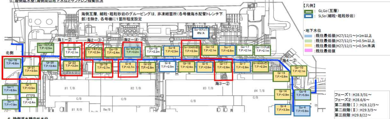
陸側遮水壁運用における監視項目（海側 互層、細粒・粗粒砂岩層水頭）
