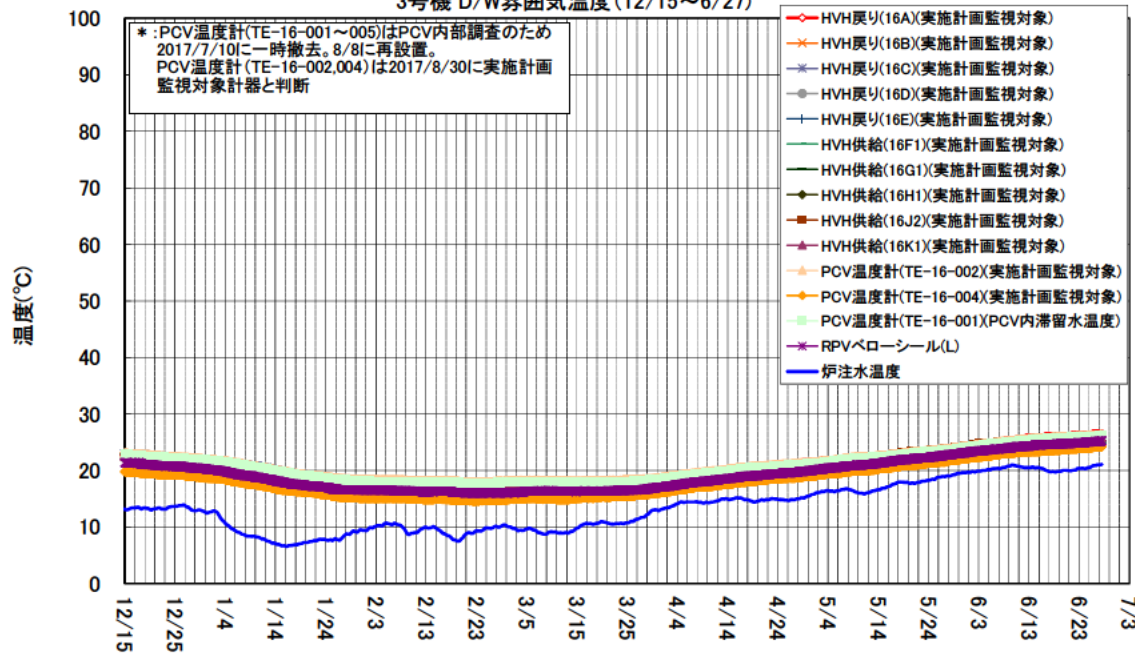
3号機 D/W雰囲気温度(12/15~6/27)
