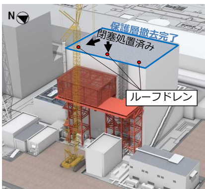
2号機原子炉建屋 鳥瞰図
