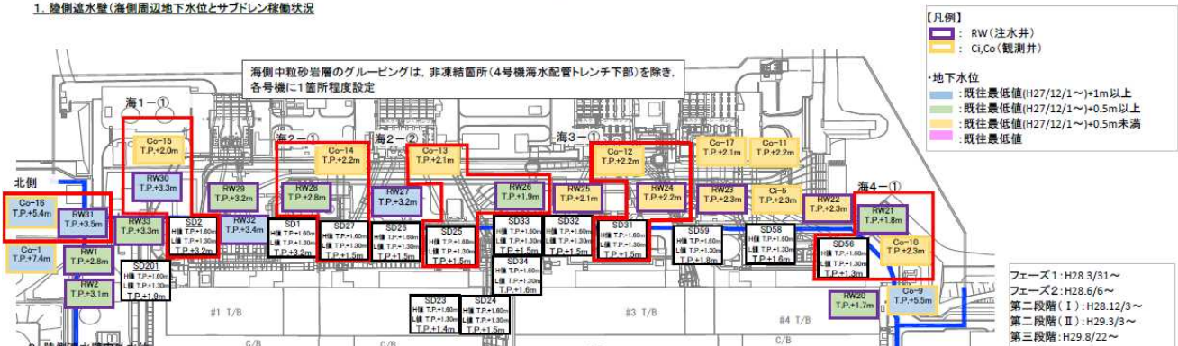
陸側遮水壁運用における監視項目(海側 中粒砂岩層水位)
