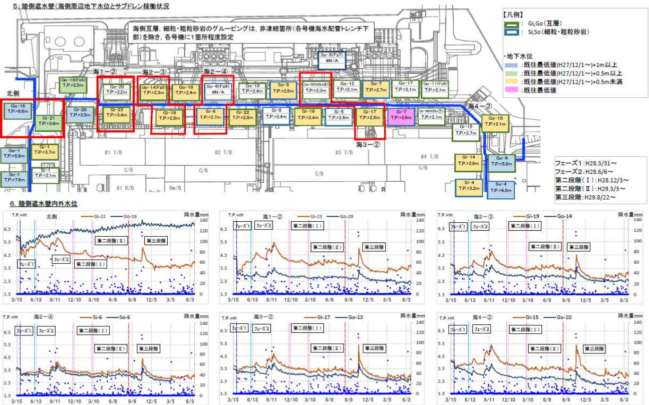
陸側遮水壁運用における監視項目（海側 互層、細粒・粗粒砂岩層水頭）
