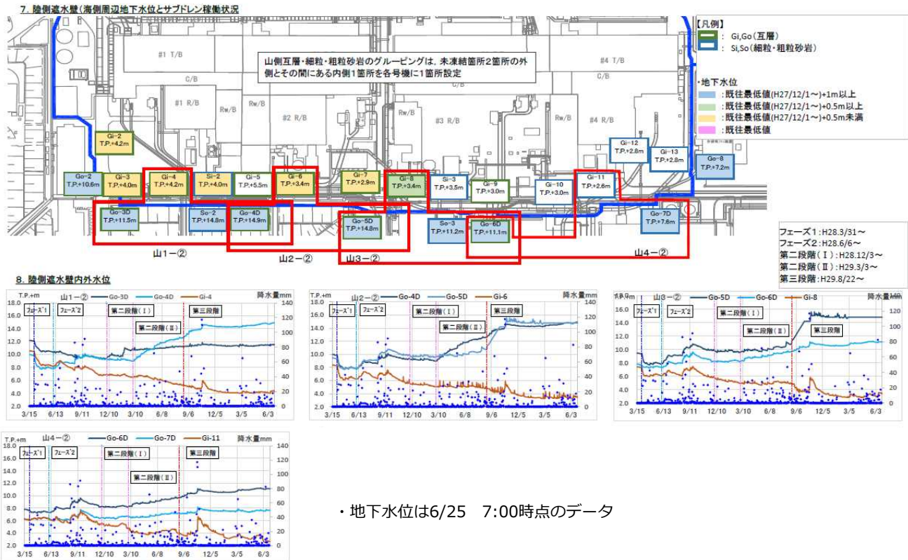
陸側遮水壁運用における監視項目(山側 互層・細粒・粗粒砂岩水位)
