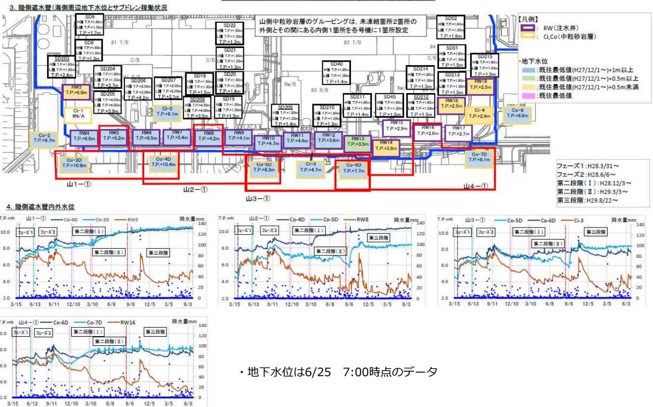
陸側遮水壁運用における監視項目（山側 中粒砂岩層水位）
