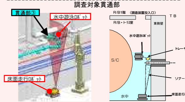
トラス室東側断面調査イメージ
