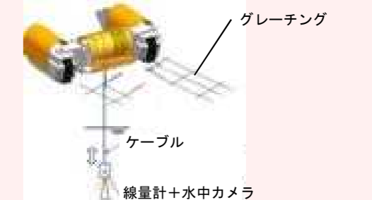
線量計、カメラ吊り降ろしイメージ
