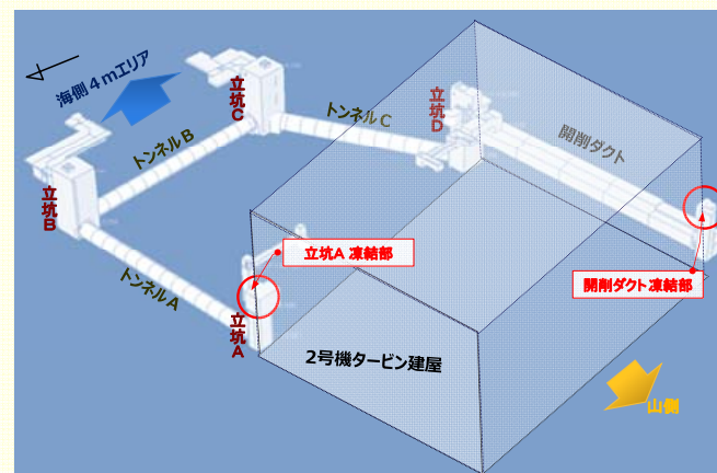
<2号機海水配管トレンチ イメージ図>
