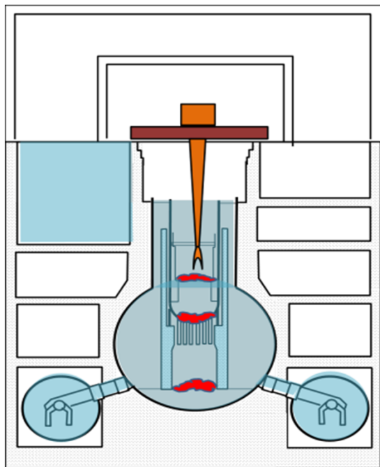
冠水-上アクセス工法
