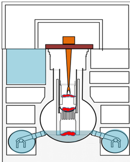
気中-上アクセス工法
