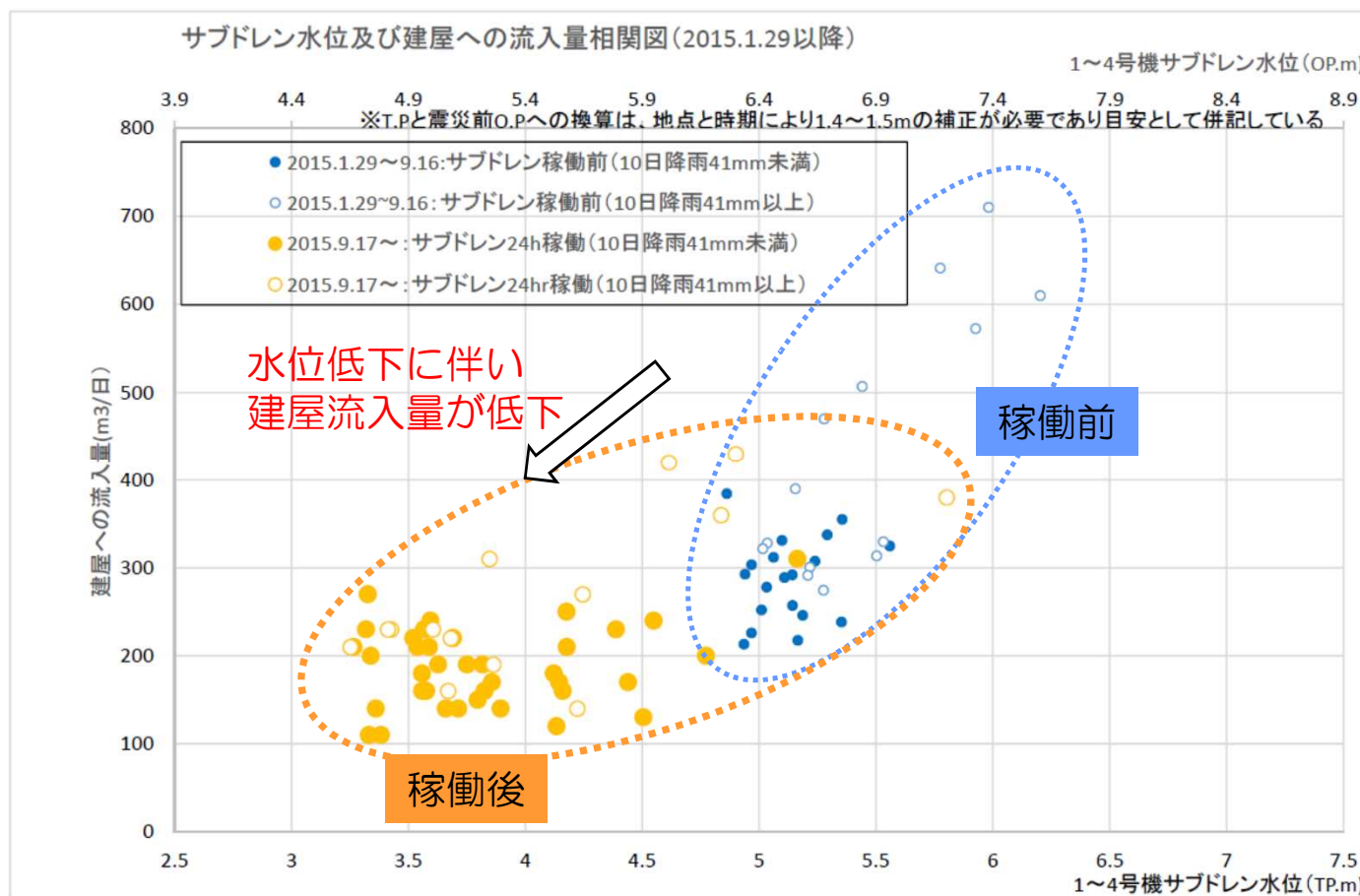
サブドレン平均水位ー建屋流入量
