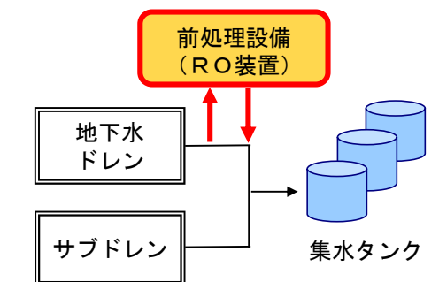
④地下水ドレン前処理設備
