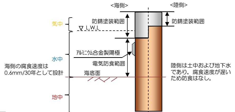
【鋼管矢板の防食イメージ】
