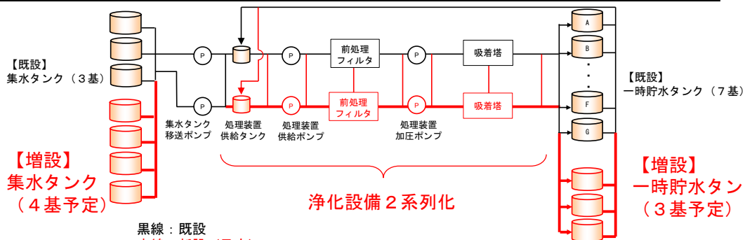
③サブドレン他浄化設備 増強イメージ
