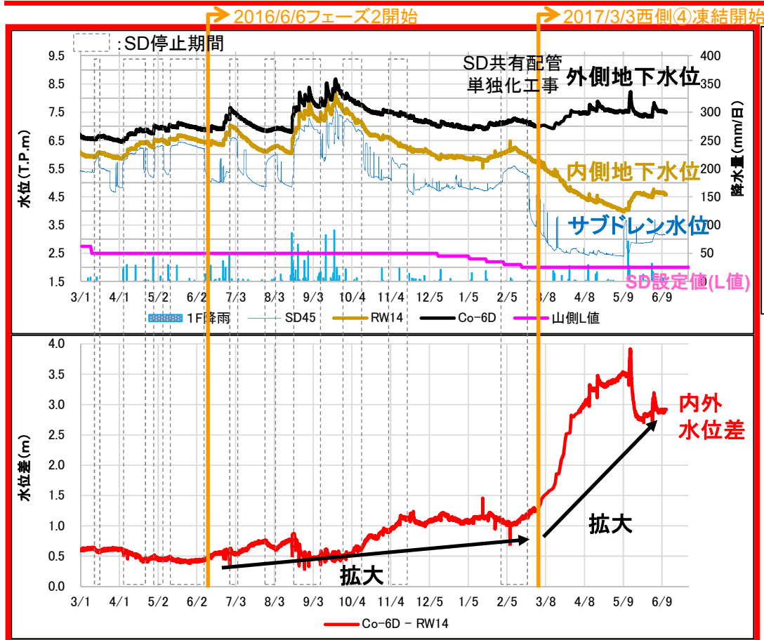
山側の内外水位挙動と水位差（#3R/B山側）
