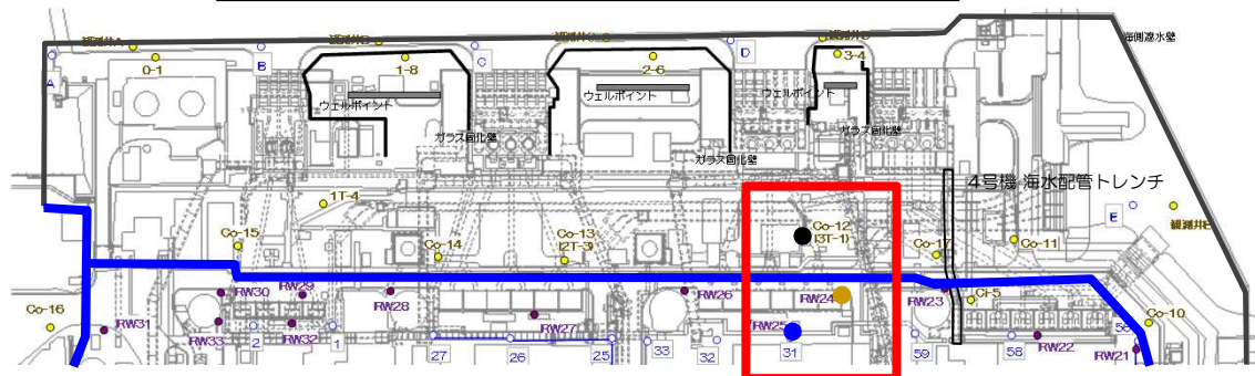
海側の内外水位挙動と水位差（#3T/B海側）
