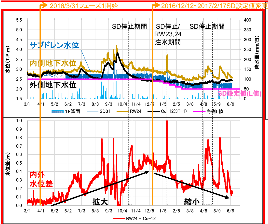
海側の内外水位挙動と水位差（#3T/B海側）
