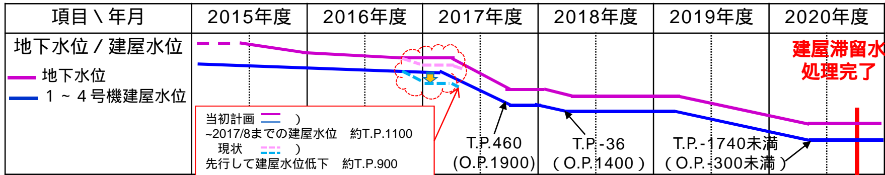
建屋滞留水の水位低下実績及び今後の計画
