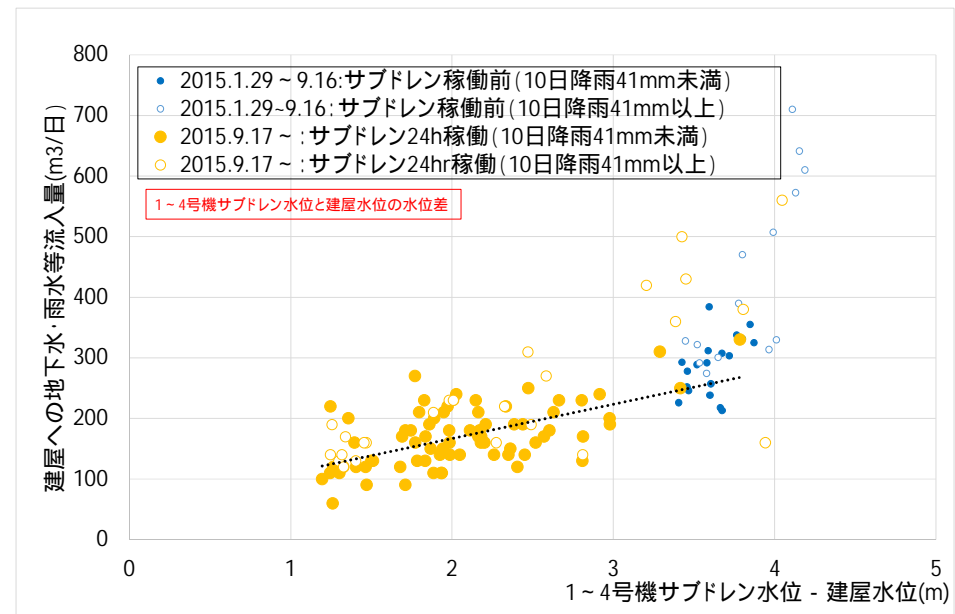
建屋内外水位差と地下水・雨水等流入量の相関
