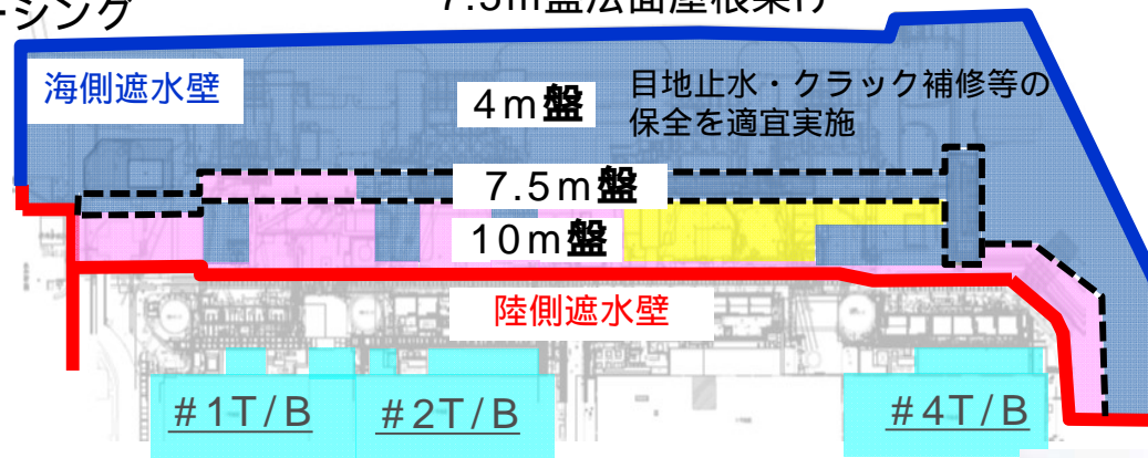
7.5m盤法面屋根架け
