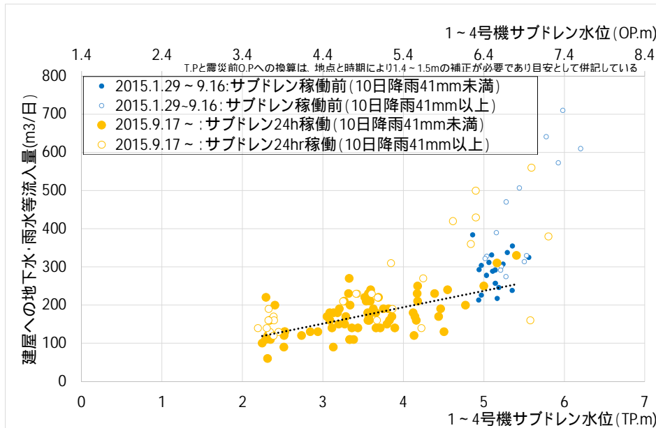
サブドレン水位と地下水・雨水等流入量の相関
