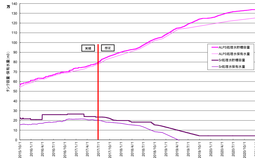
タンク建設の見通し (サブドレン + 陸側遮水壁)
