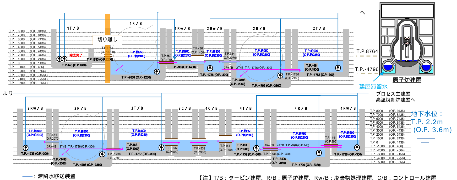
1～4号機の建屋床面レベル、建屋間貫通部及び滞留水の水位(2017.8.16時点)
