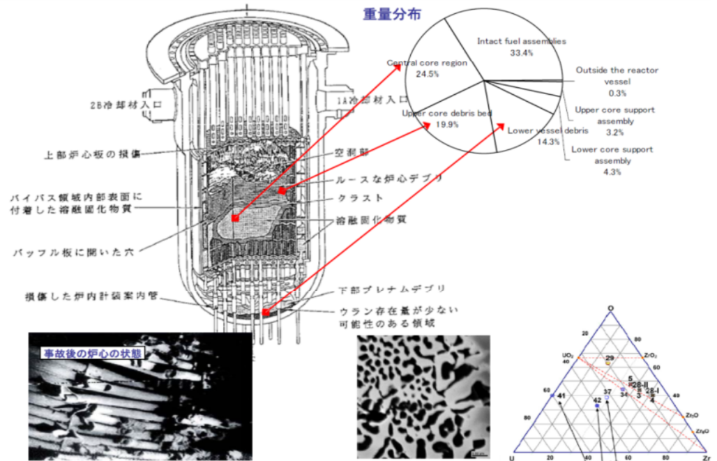
図 TMI事故時の炉心の状況
