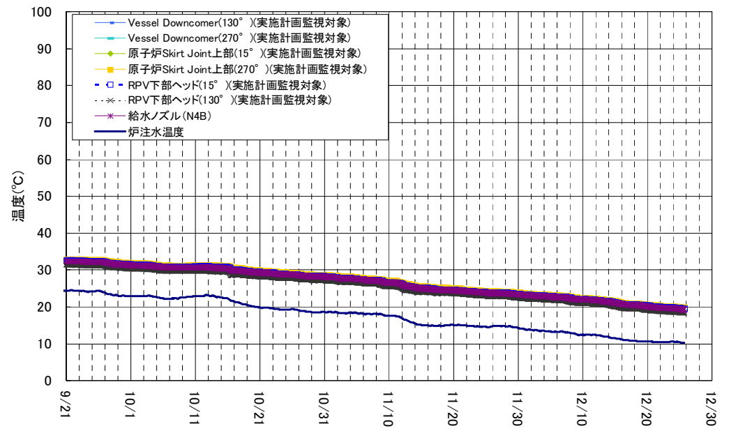
1号機 原子炉圧力容器まわり温度 (9/21~12/25)
