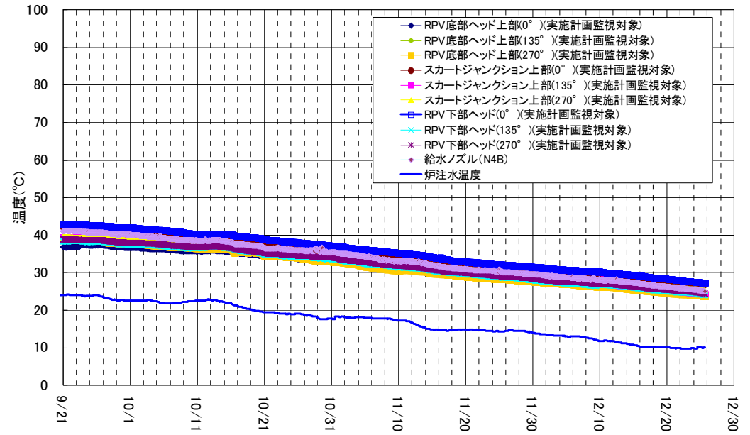
3号機 原子炉圧力容器まわり温度 (9/21~12/25)
