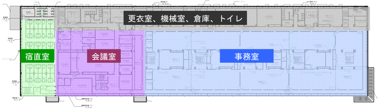
2階平面図
