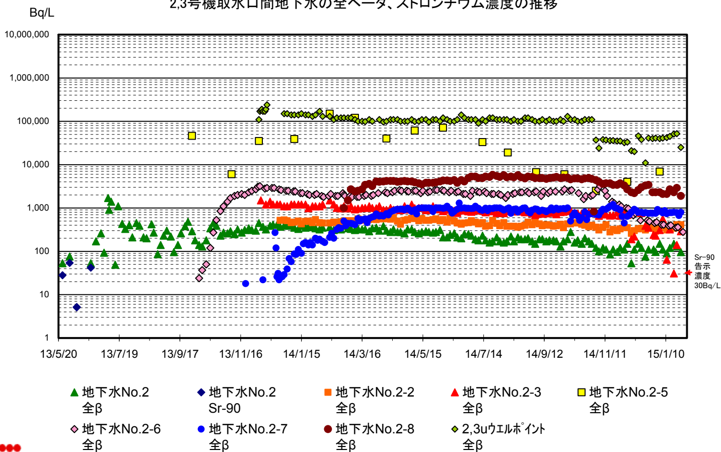
2,3号機取水口間地下水の全ベータ、ストロンチウム濃度の推移
