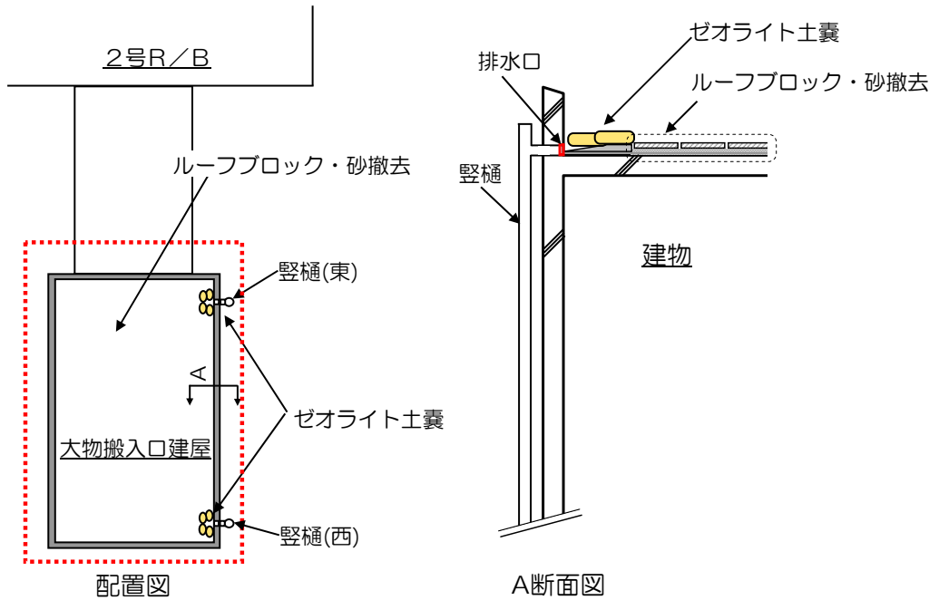
ゼオライト土嚢 設置イメージ
