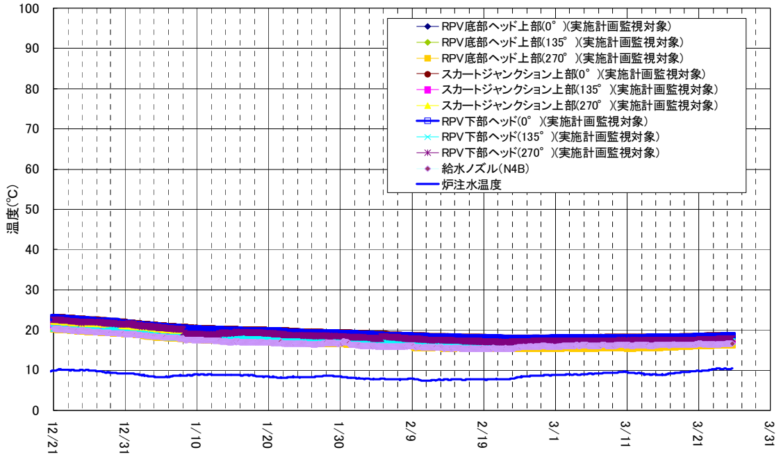
3号機 原子炉圧力容器まわり温度 (12/21~3/25)
