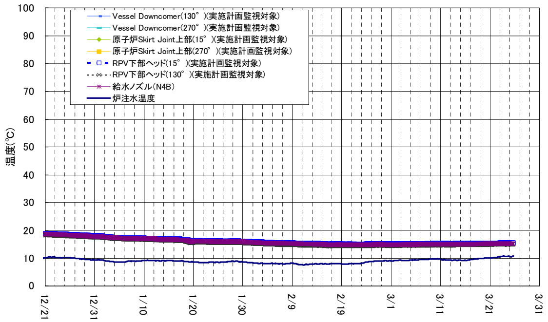
1号機 原子炉圧力容器まわり温度 (12/21~3/25)
