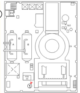
4階 平面図
