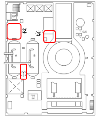
4階 平面図
