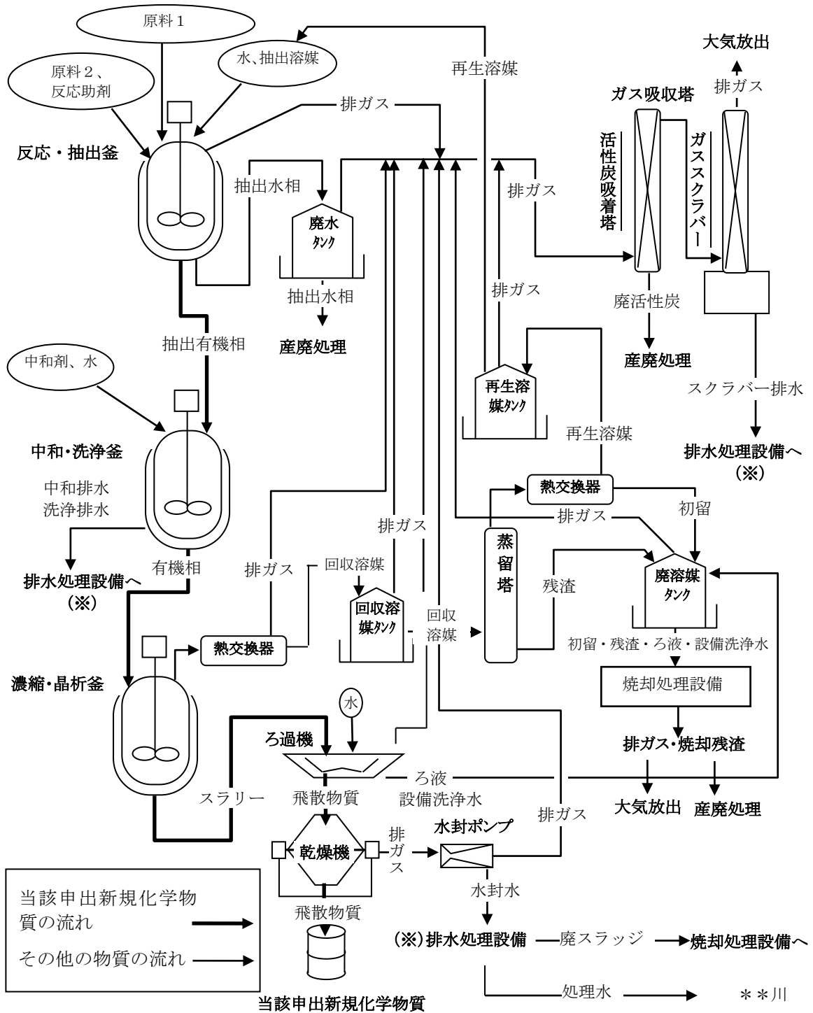
② 製造設備の状況を示す図面
