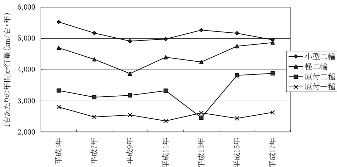
図 13-15 車種別の二輪車1台あたりの走行量
