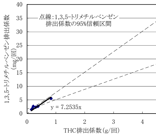
図 12-42 ガソリン自動車(コールドスタート時の増分)に係る THC 排出量と対象化学物質別排出量の比率(その1)
