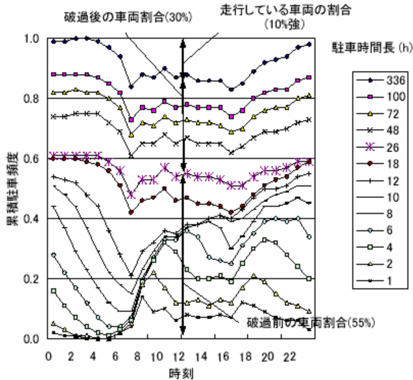
図 12-47 時刻ごとの駐車時間長別車両数構成比(自家用乗用車の例)
