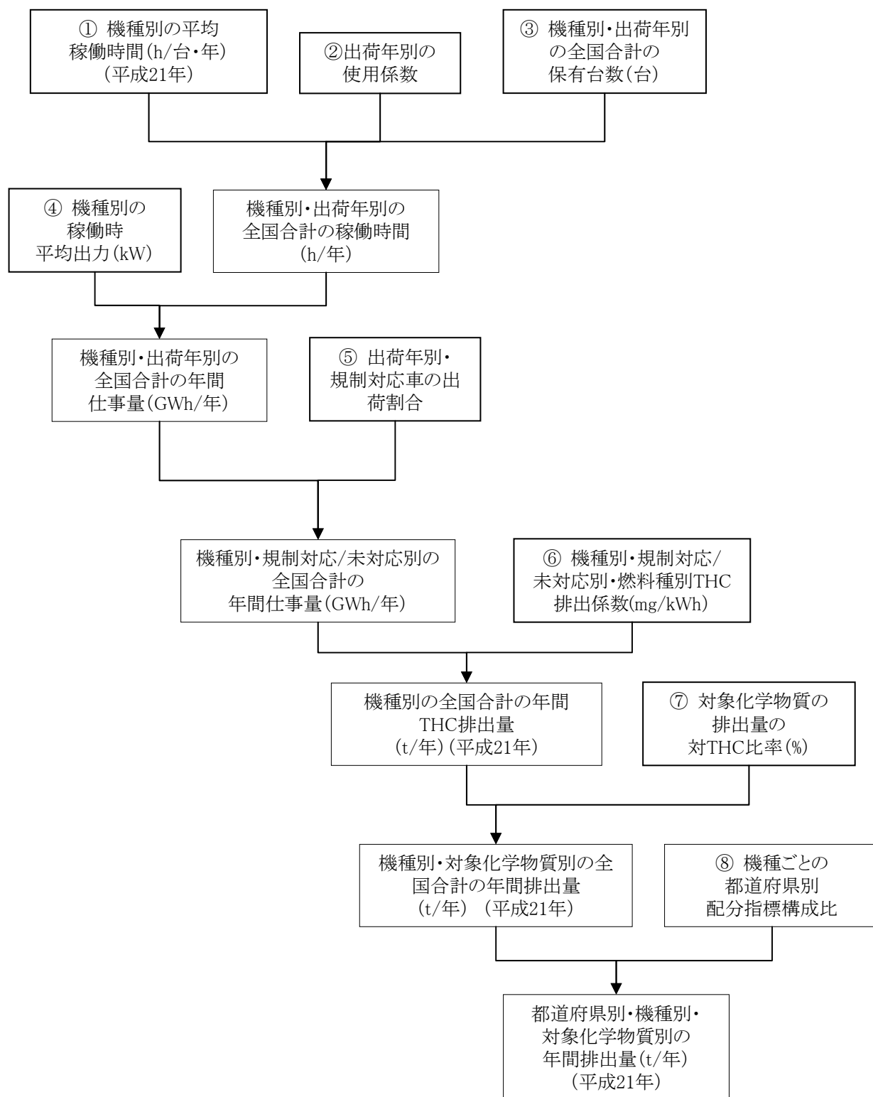
図 12-37 自動車(サブエンジン式機器)に係る排出量の推計フロー
