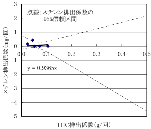
図 12-43 ディーゼル自動車(コールドスタート時の増分)に係る THC 排出量と対象化学物質別排出量の比率(その1)
