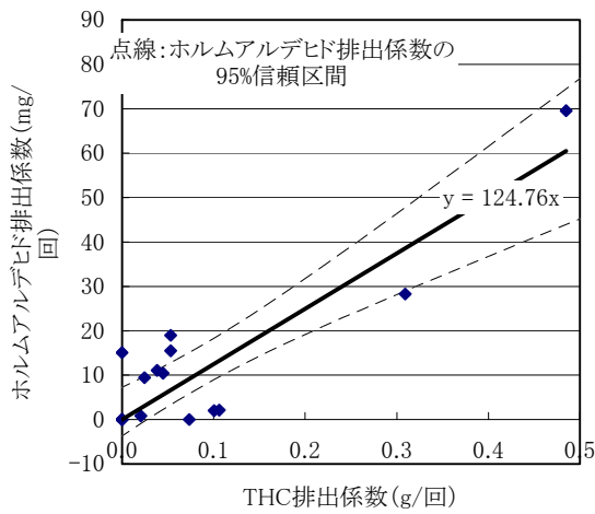
図 12-43 ディーゼル自動車(コールドスタート時の増分)に係るTHC排出量と対象化学物質別排出量の比率(その2)
