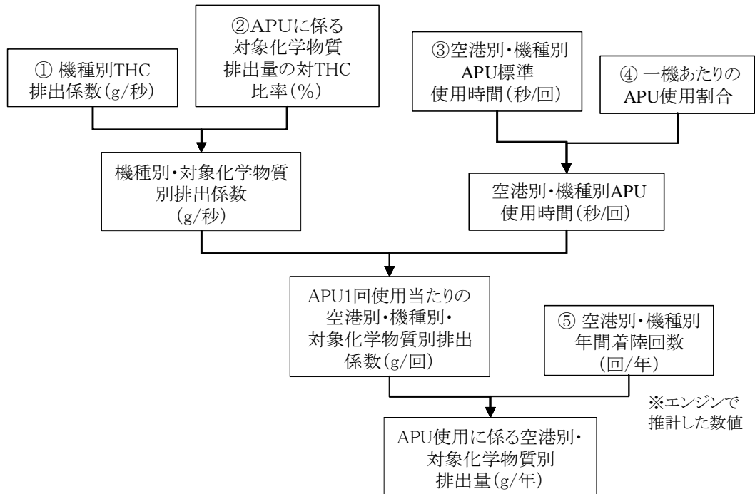
図16-4 補助動力装置 (APU) に係る排出量の推計フロー
