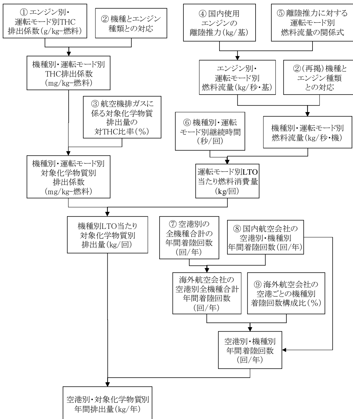
図16-3 航空機(エンジン)に係る排出量の推計フロー
