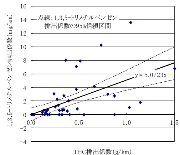
図11-39 ディーゼル自動車(ホットスタート:重量車)に係る THC 排出量と対象化学物質別排出量の比率(その1)
