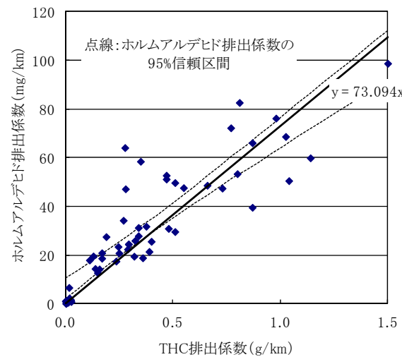
図11-39 ディーゼル自動車(ホットスタート:重量車)に係る THC 排出量と対象化学物質別排出量の比率(その2)
