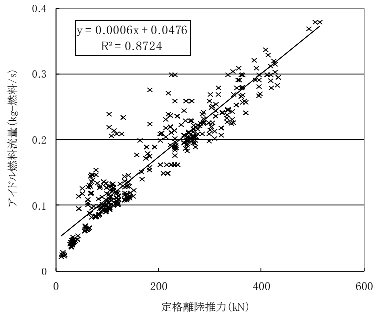
図 16-2 定格離陸推力と燃料流量の関係(アプローチ及びアイドル)
