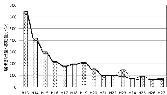
1,3-ブタジエン(351)
