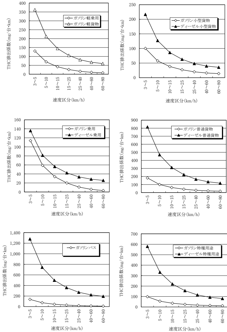
図11-13 車種別・旅行速度区分別の THC 排出係数(平成 27 年度;触媒の劣化補正後)
