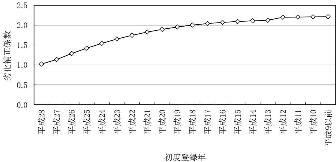
図11-11 初度登録年別の劣化補正係数の推計結果(平成27年度;ガソリン乗用車の例)
